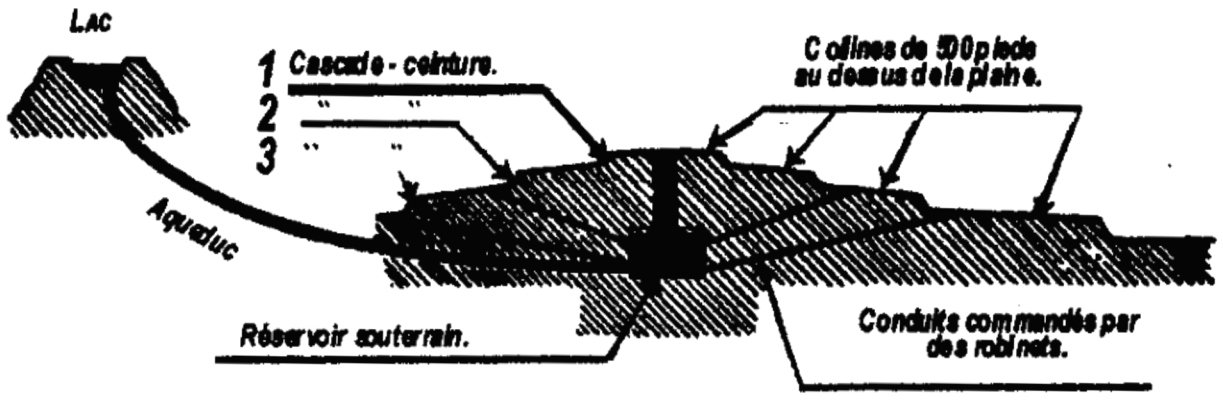
— DISTRIBUTION D'EAU (VUE EN COUPE) —
